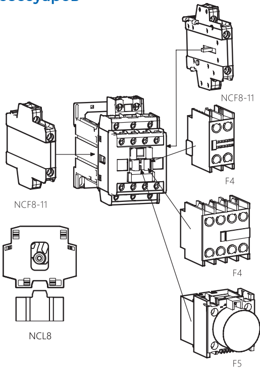
Контактор NC8 с аксессуарами
